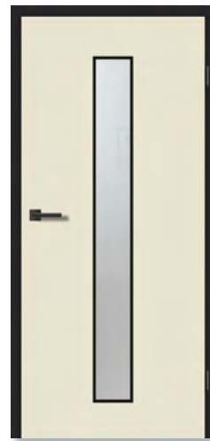
TB-LA2 mittig G-TEC® LiveSimple matt CN08 Glas Float satiniert Glasleisten G-TEC® Schwarz matt FU G-TEC® Schwarz matt 9005 Beschlag LUCIA PIATTA S QUATTRO Graphitschwarz smart2lock ohne Schlüssellochbohrung
