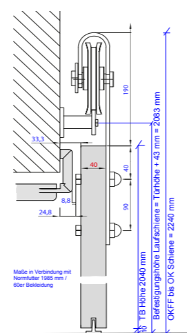
Außenlaufend, mit Futter
